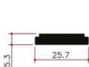
Y11311 0.348Kg/m
