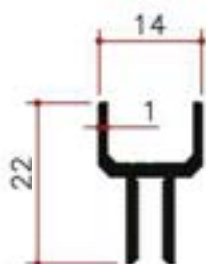
Y13998 0.186Kg/m
