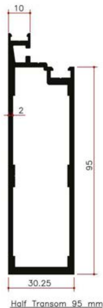
Y23206 1.731Kg/m
