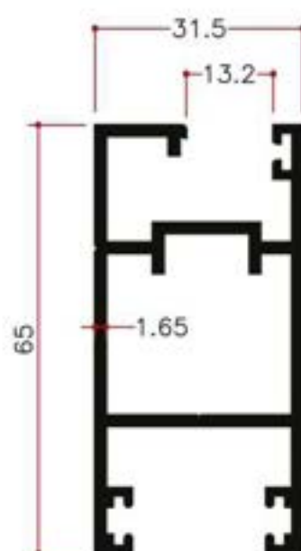
Y24881 1.066Kg/m
