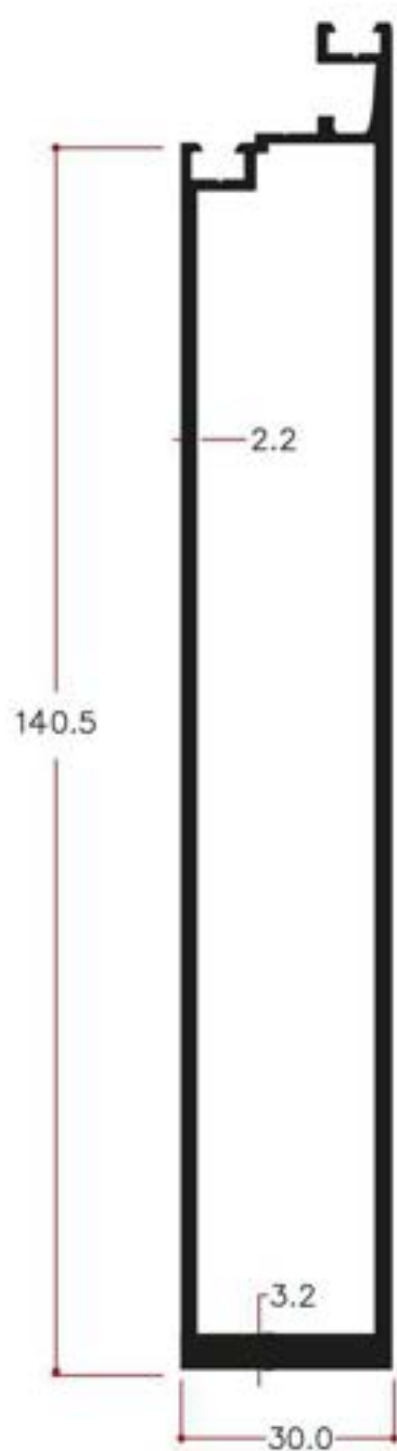
Y1808 2.287 Kg/m
