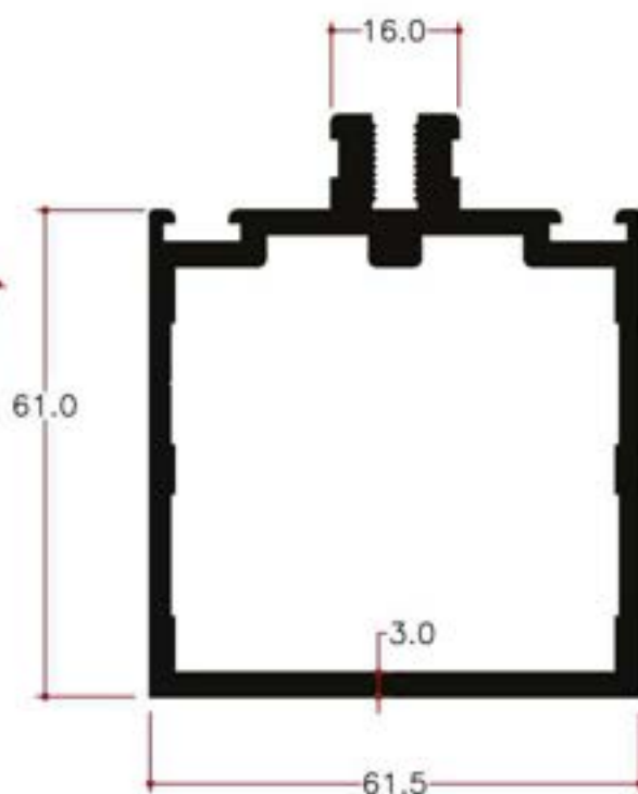
Y23459 2.234Kg/m
