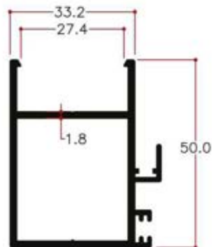
Y22468 0.888Kg/m
