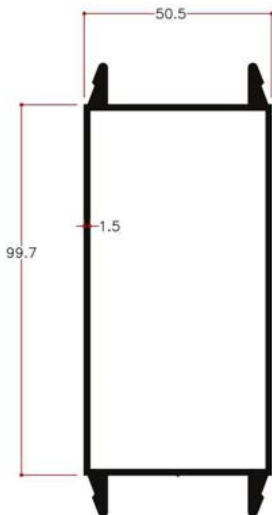
Y24449 1.626Kg/m
