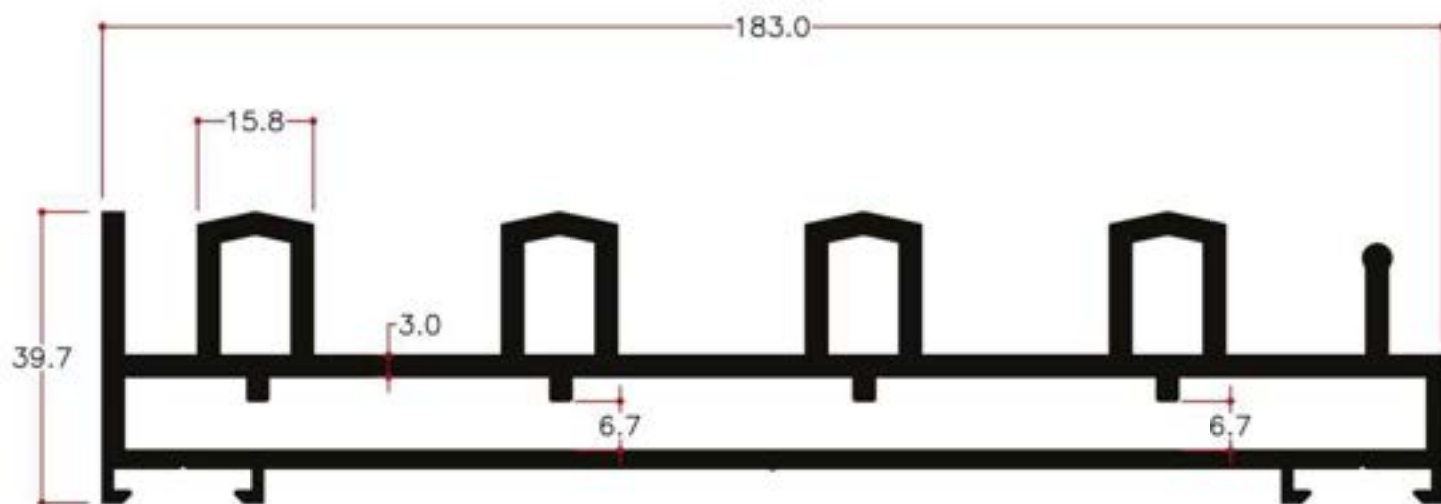
Y26384 4.861Kg/m
