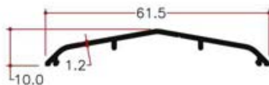
Y13606 0.241Kg/m
