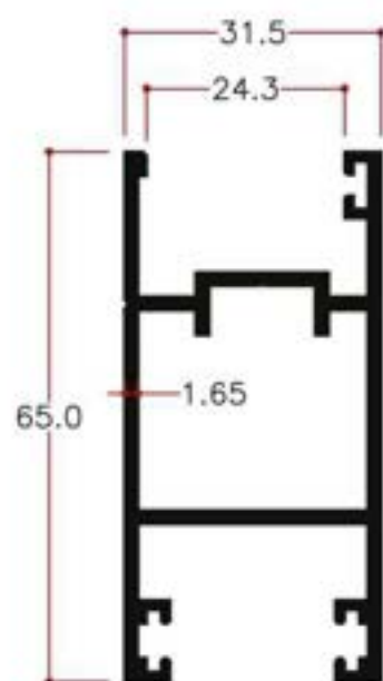
Y24880 1.007Kg/m
