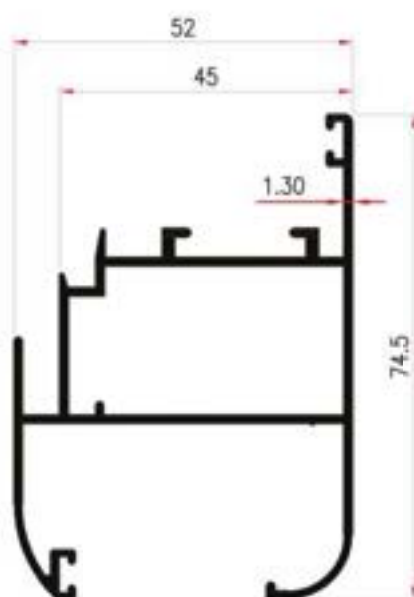
Y25078 ( 1.016 Kg/m)
