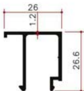
Y12285 0.289Kg/m
