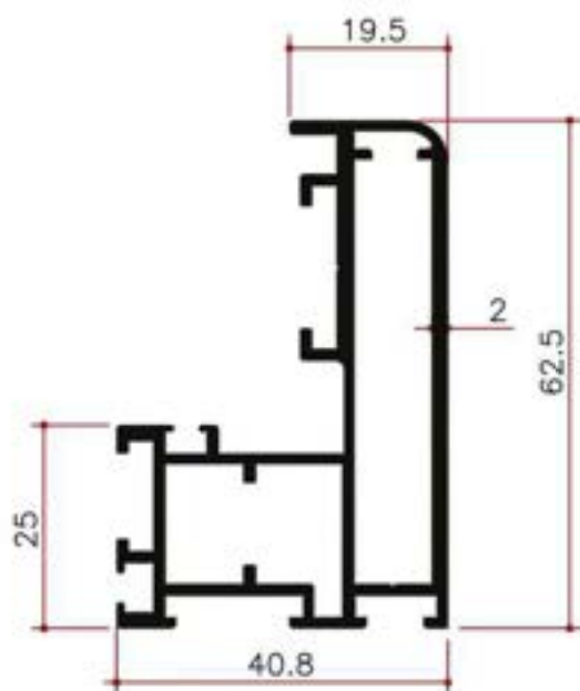
Y23407 1.222Kg/m
