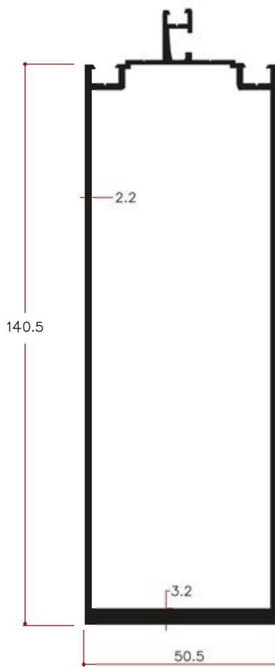
Y1807 2.443 Kg/m
