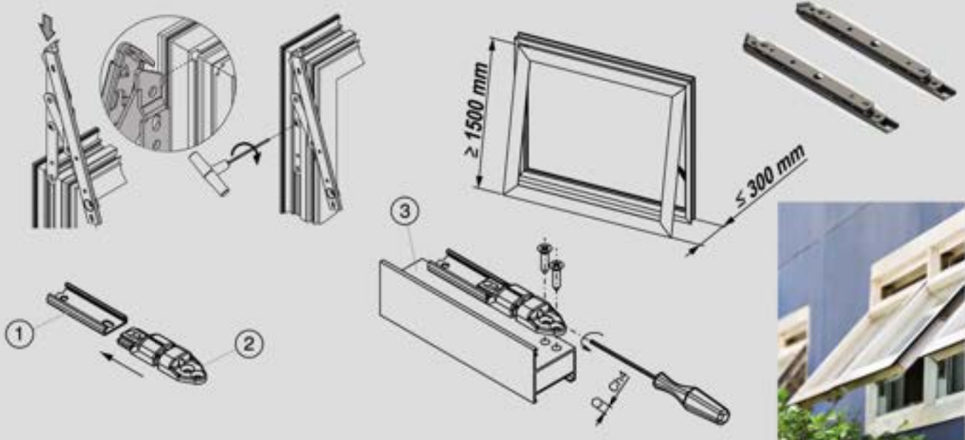
Unica cremone
