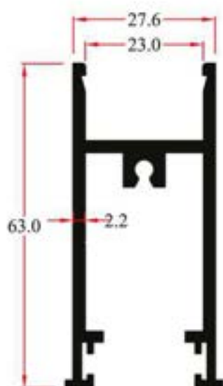
Y13768 1.033Kg/m
