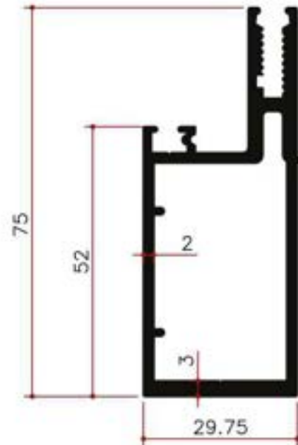
Y25091 1.303Kg/m
