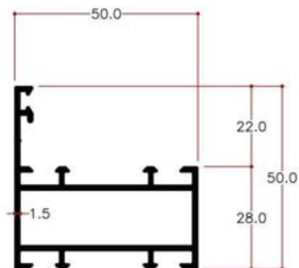
Y26483 0,889 Kg/m
