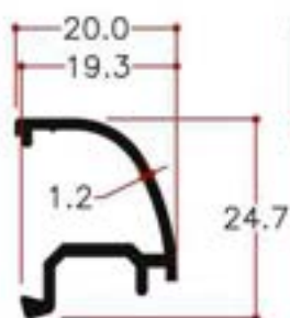
Y12413 0.222Kg/m
