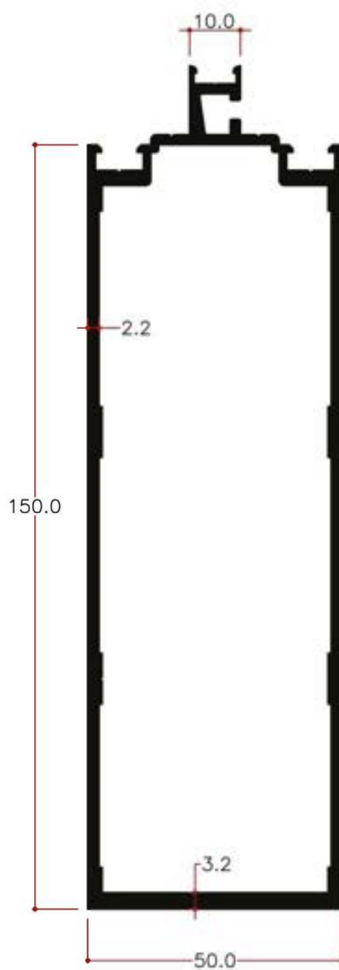
Transom 150 mm
