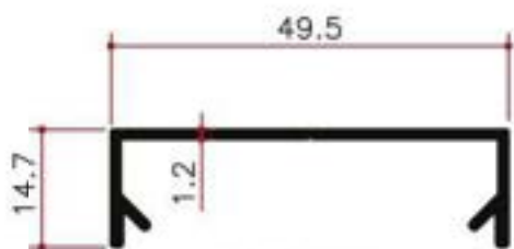
Y13983 0.287Kg/m
