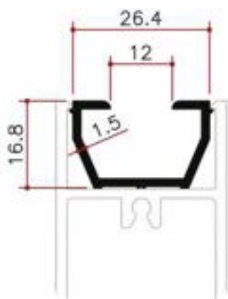
Y14719 0.254Kg/m
