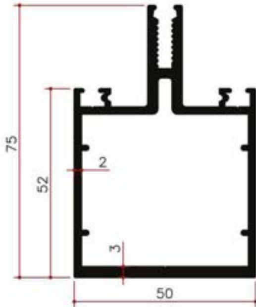
Y24362 1.649Kg/m
