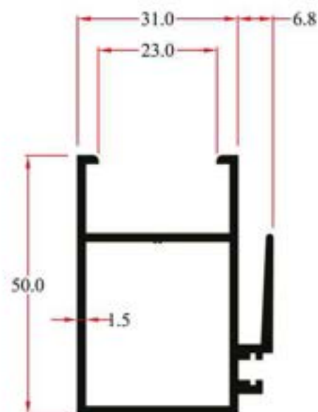
Y24651 0.816Kg/m
