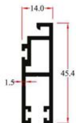
Y26211 0.539Kg/m
