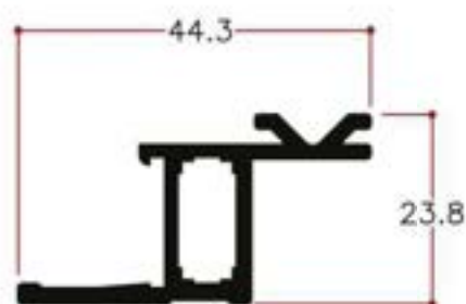
Str. Vent frame adator
