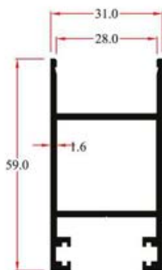
Y25314 0.812Kg/m
