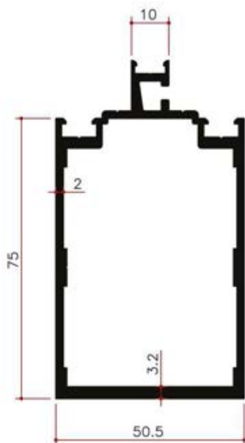
Transom 75 mm
