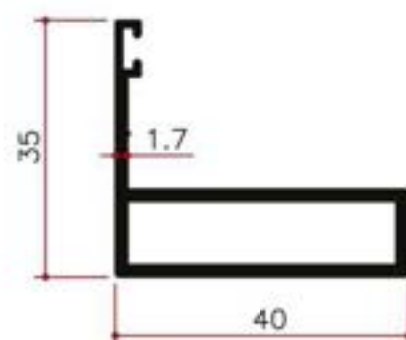
Y24804 0.557Kg/m
