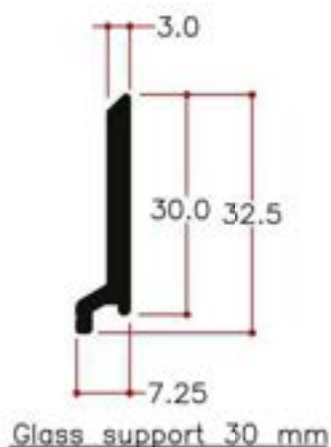
Y12896 0.268Kg/m
