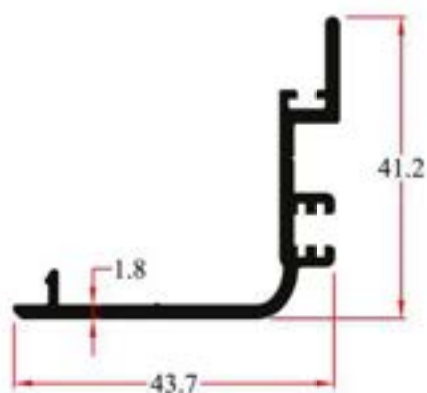
Y15857 0.484Kg/m
