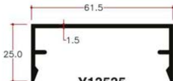
Y13535 0.496Kg/m
