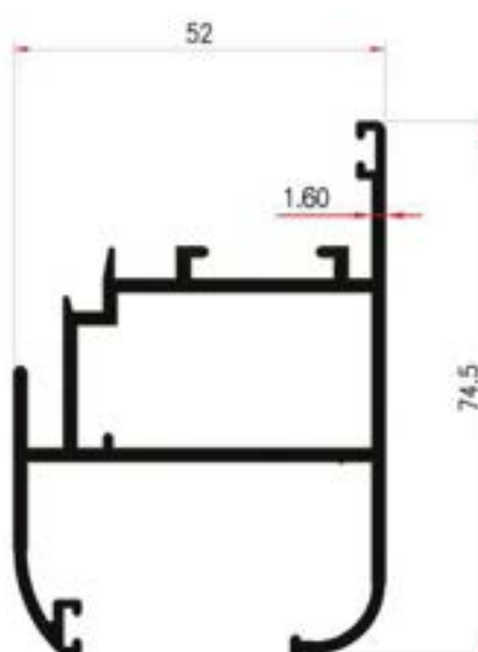
Y6535 ( 1.186 Kg/m)
