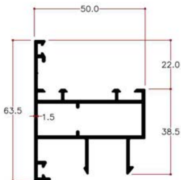
Y26454 1,038 Kg/m
