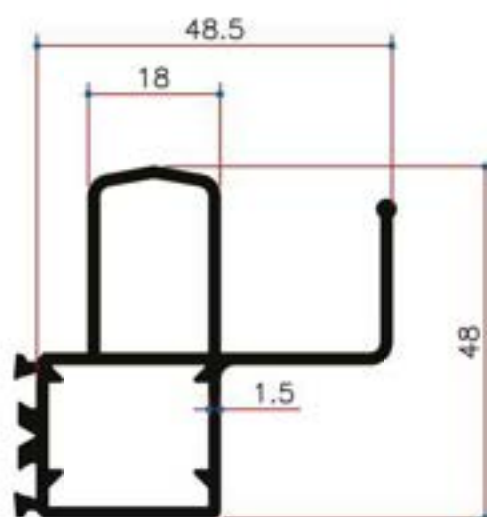
Y23017 0.898Kg/m
