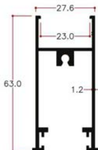
Y12123 0.699Kg/m
