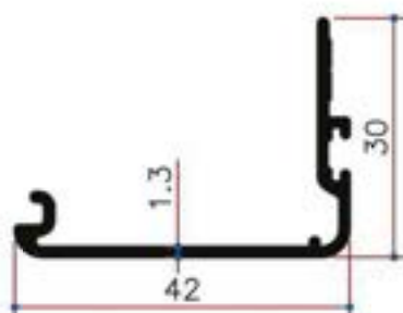
Y13066 0.316Kg/m
