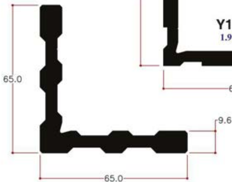
Y11672 2.447Kg/m
