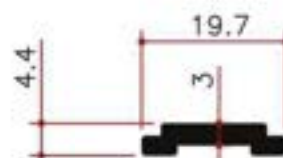
Y11241 0.172Kg/m
