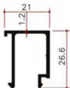
Y12284 0.273Kg/m
