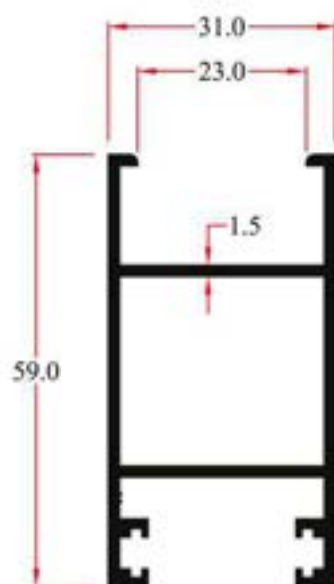
Y24650 0.811Kg/m
