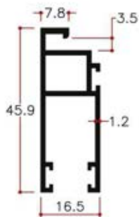
Y21649 0.441Kg/m
