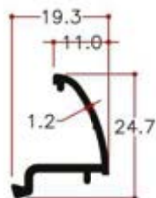
Y11743 0.185Kg/m
