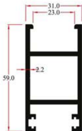
Y23964 1.085Kg/m
