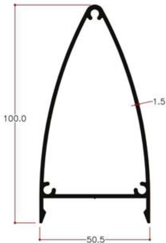
Y24448 1.139Kg/m
