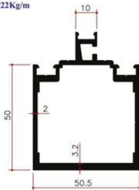
Transom 50 mm
