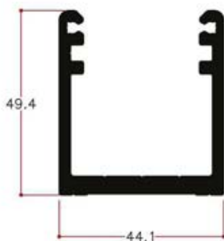
Y11674 1.444Kg/m
