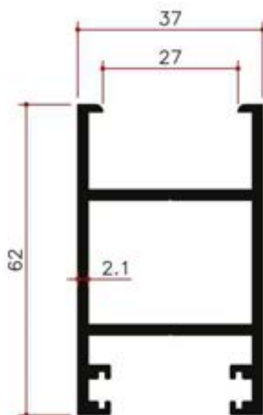
Y24917 1.202Kg/m
