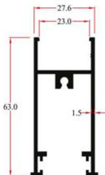
Y11613 0.807Kg/m
