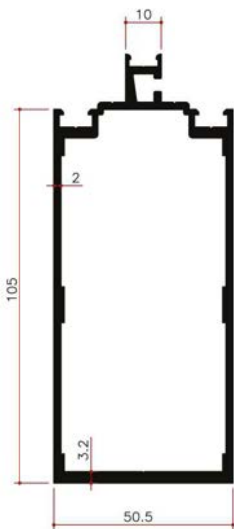
Transom 105 mm
