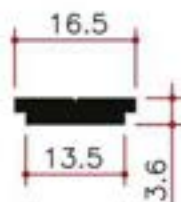
Y13329 0.147Kg/m
