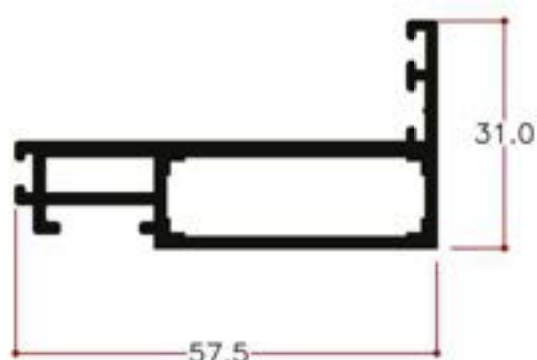
Str. Vent frame
