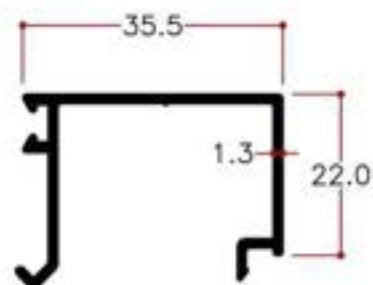
Y16055 0,349 Kg/m
