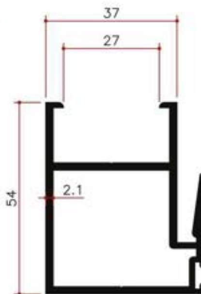
Y24918 1.188Kg/m
