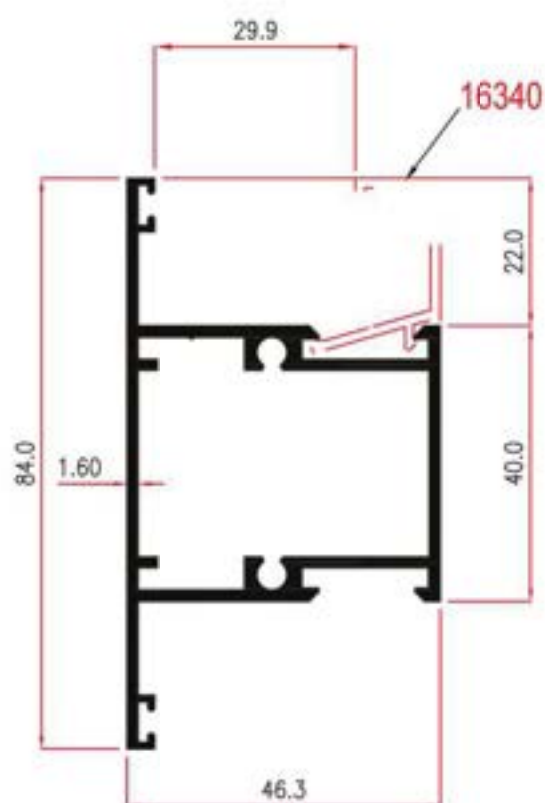
Y24992 1.218 Kg/m
