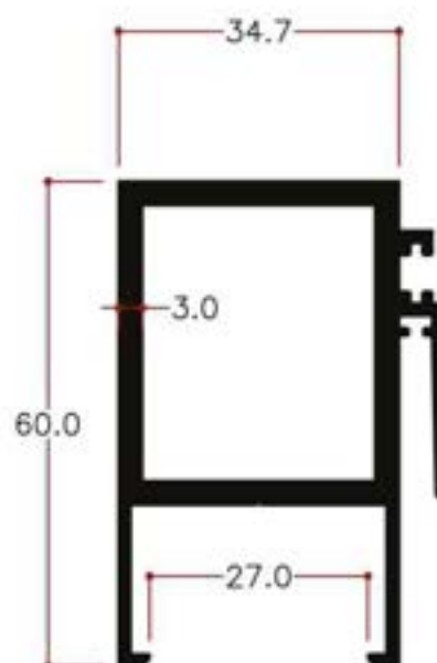
Y24727 1.428Kg/m
