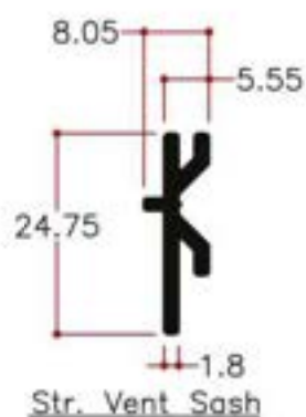
Y12902 0.203Kg/m
