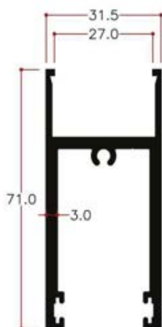
Y14879 1.253Kg/m
