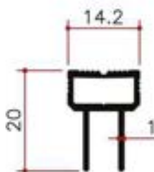
Y24166 0.179Kg/m
