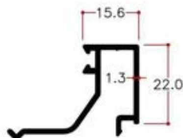
Y16054 0,332 Kg/m
