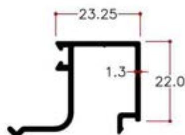
Y16090 0,338 Kg/m
