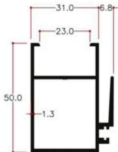
Y21651 0.746Kg/m
