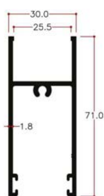
Y11205 0.921Kg/m
