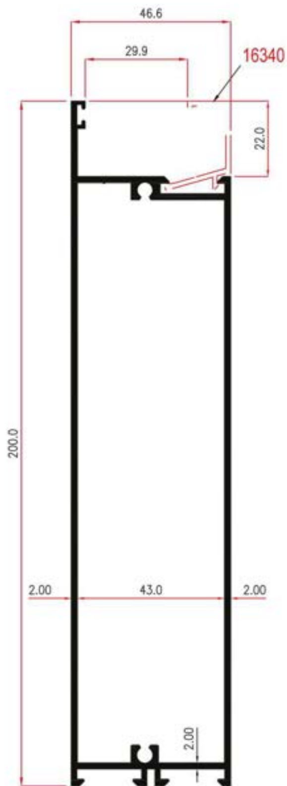
Y25850 2.310 Kg/m
