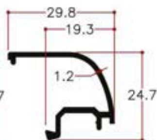
Y12650 0.254Kg/m
