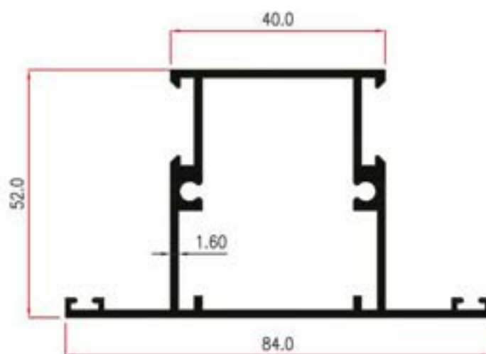
Y25852 1.260 Kg/m
