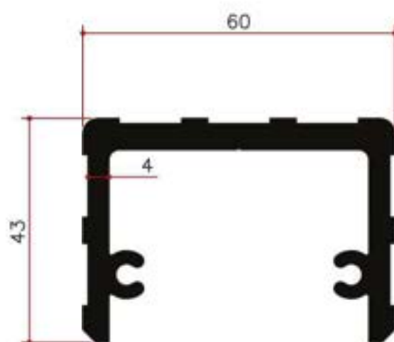
Y14910 1.924Kg/m
