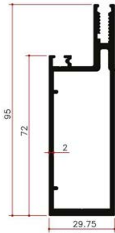
Y24365 1.525Kg/m
