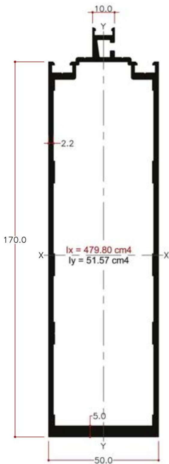
Transom 150 mm
