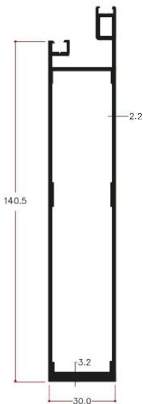
Y1806 2.380 Kg/m
